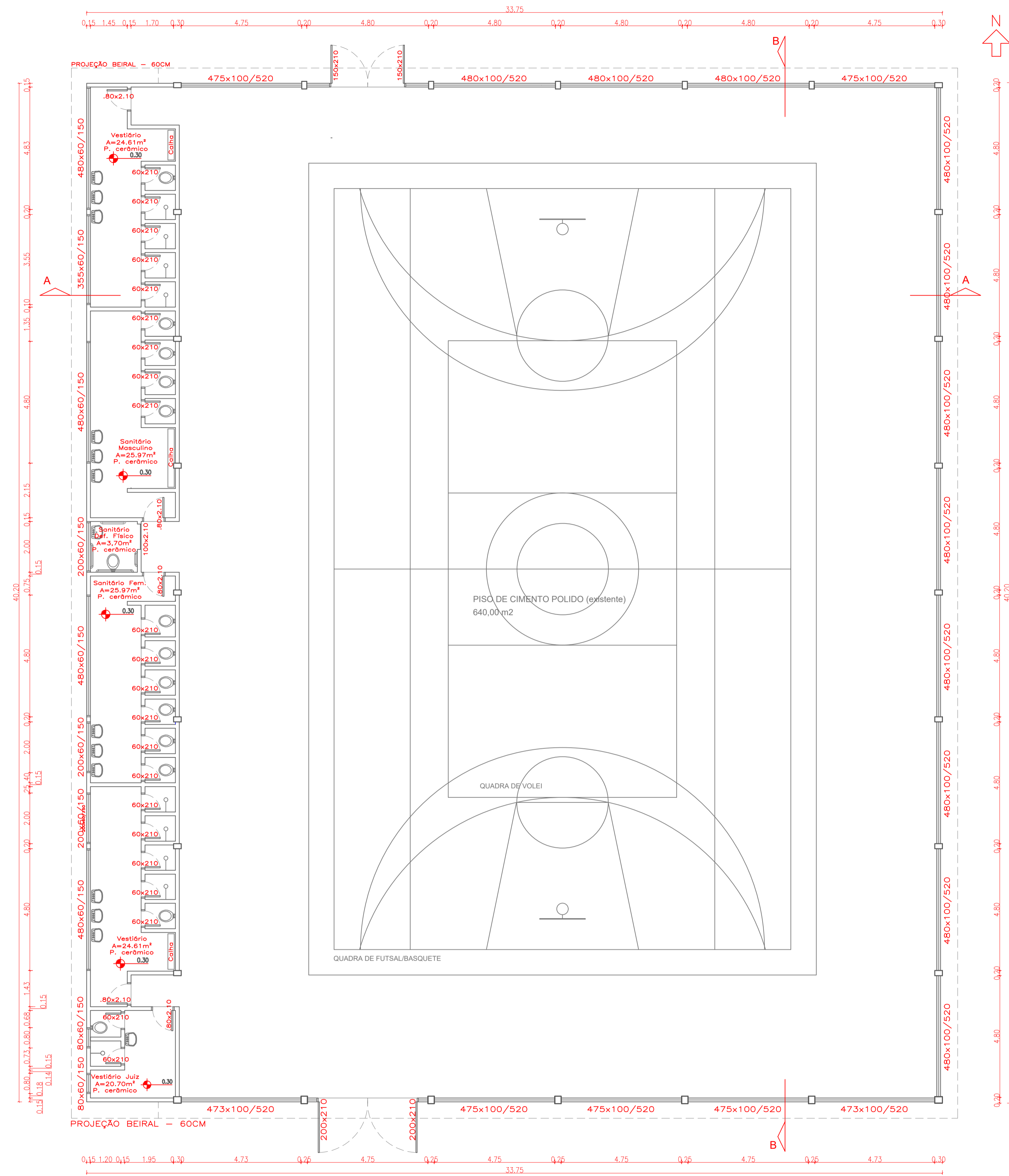
PLANTA BAIXA - HOJE Esc.: 1/100
