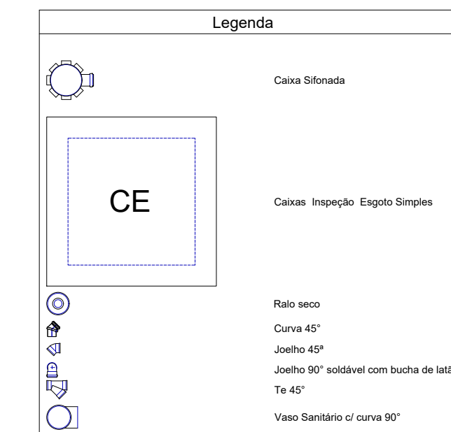
2 PLANTA VESTIÁRIO 2 ESCALA 1/25
