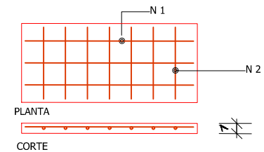
DETALHE FERRAGEM - TAMPA
