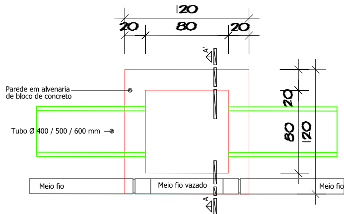
PLANTA BAIXA - CAIXA BLS (0,80 x 0,80m int.)
