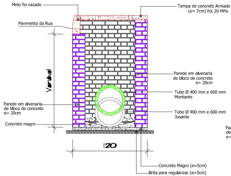
CORTE A-A' - CAIXA BLS (0,80 x 0,80m int.)
