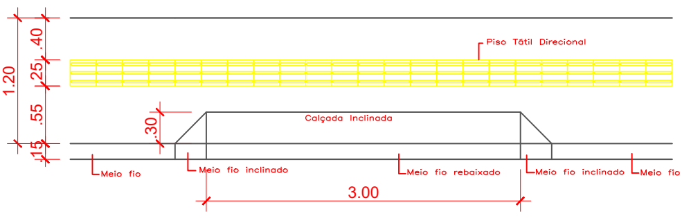
DETALHE REBAIXAMENTO MEIO FIO 02 Esc.: 1/50
