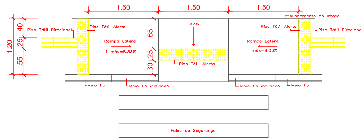
DETALHE RAMPA DE ACESSIBILIDADE Esc.: 1/50
