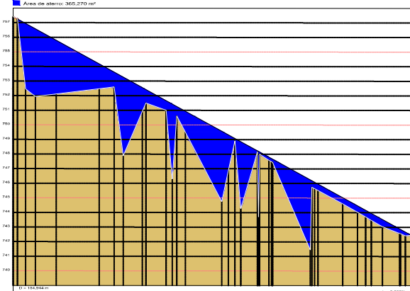
Perfil Longitudinal
