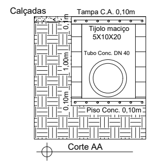
DETALHAMENTO BOCA DE LOBO Escala: 1/50
