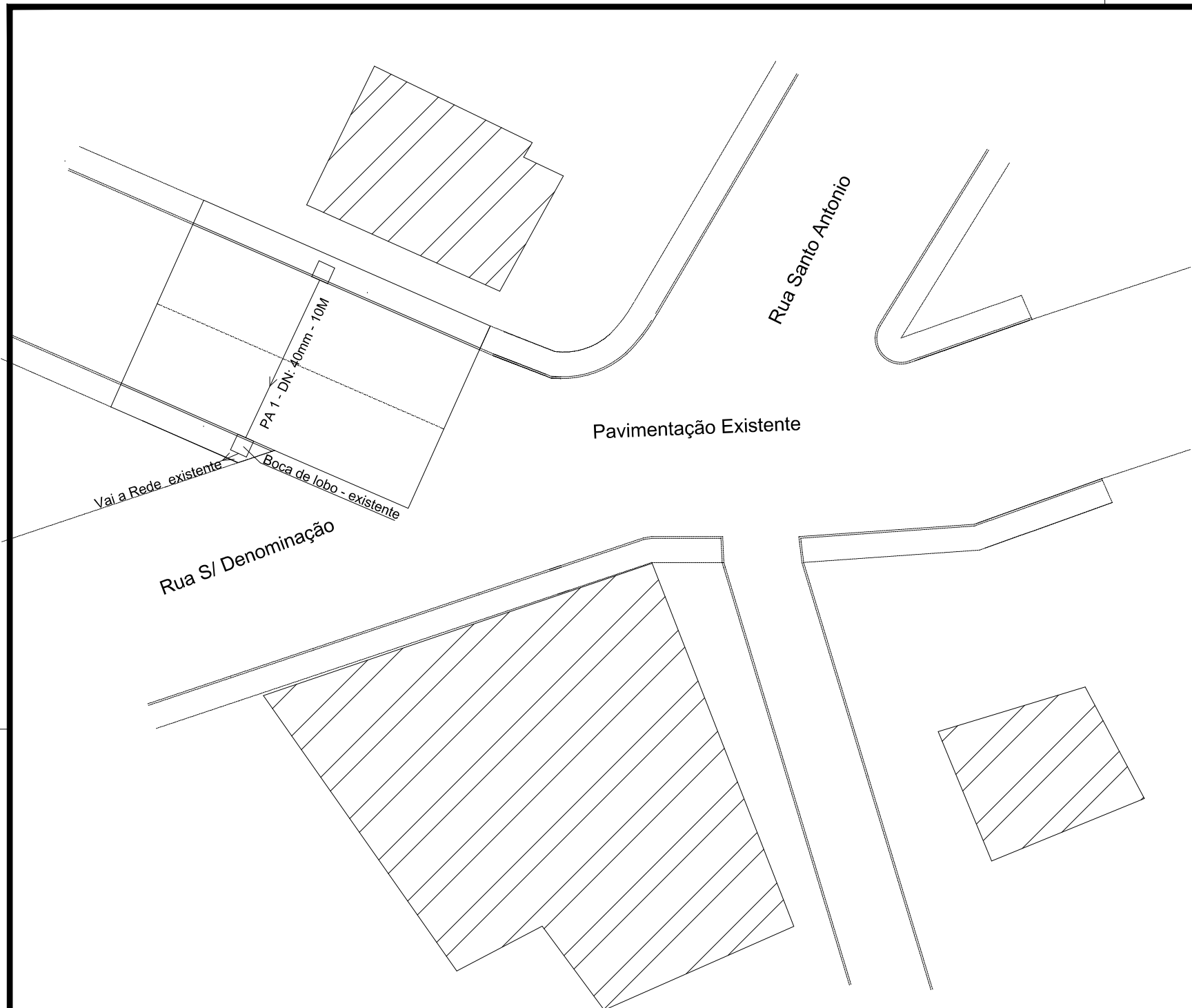
PLANTA BAIXA - DRENAGEM ESCALA: 1/300
